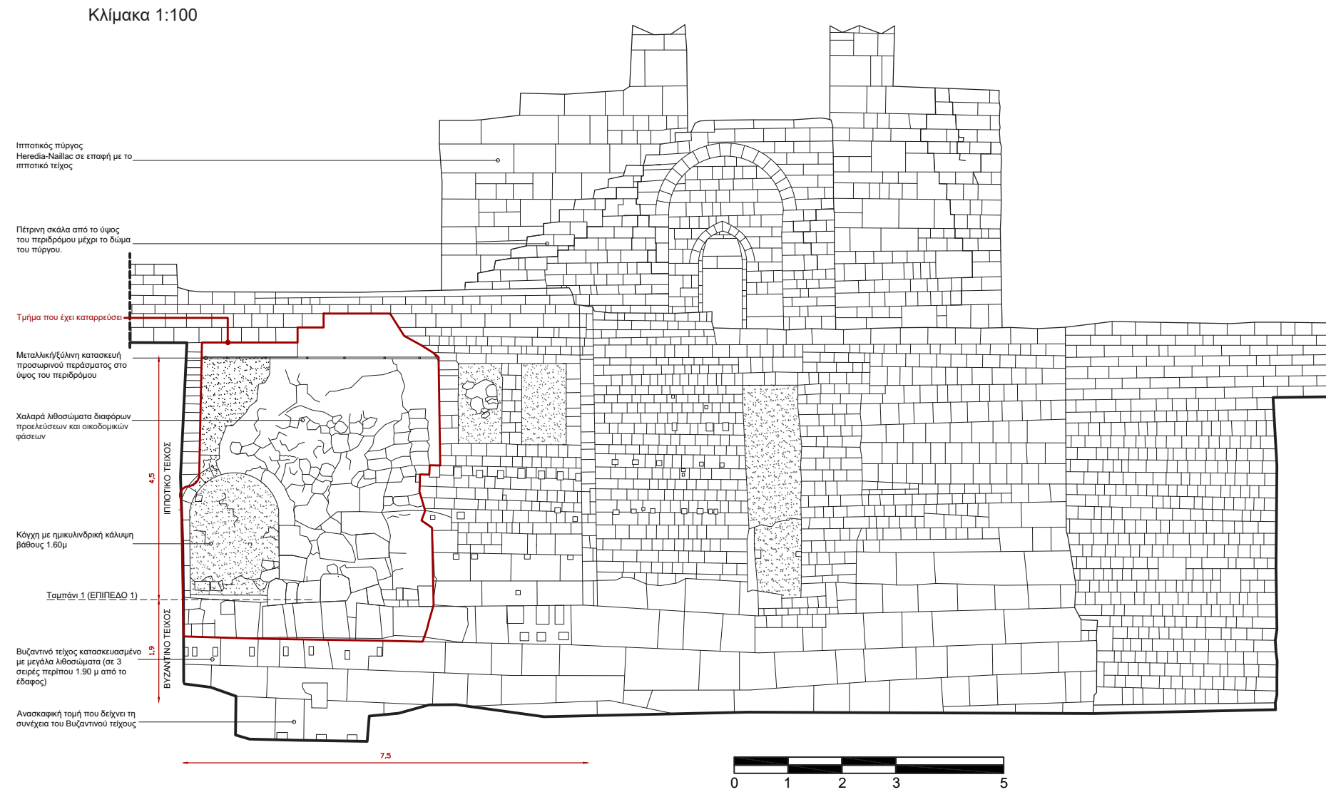
Σχ 1. Εσωτερική όψη του τείχους υφιστάμενης κατάστασης -ΜΕΤΑ την κατάρρευση
