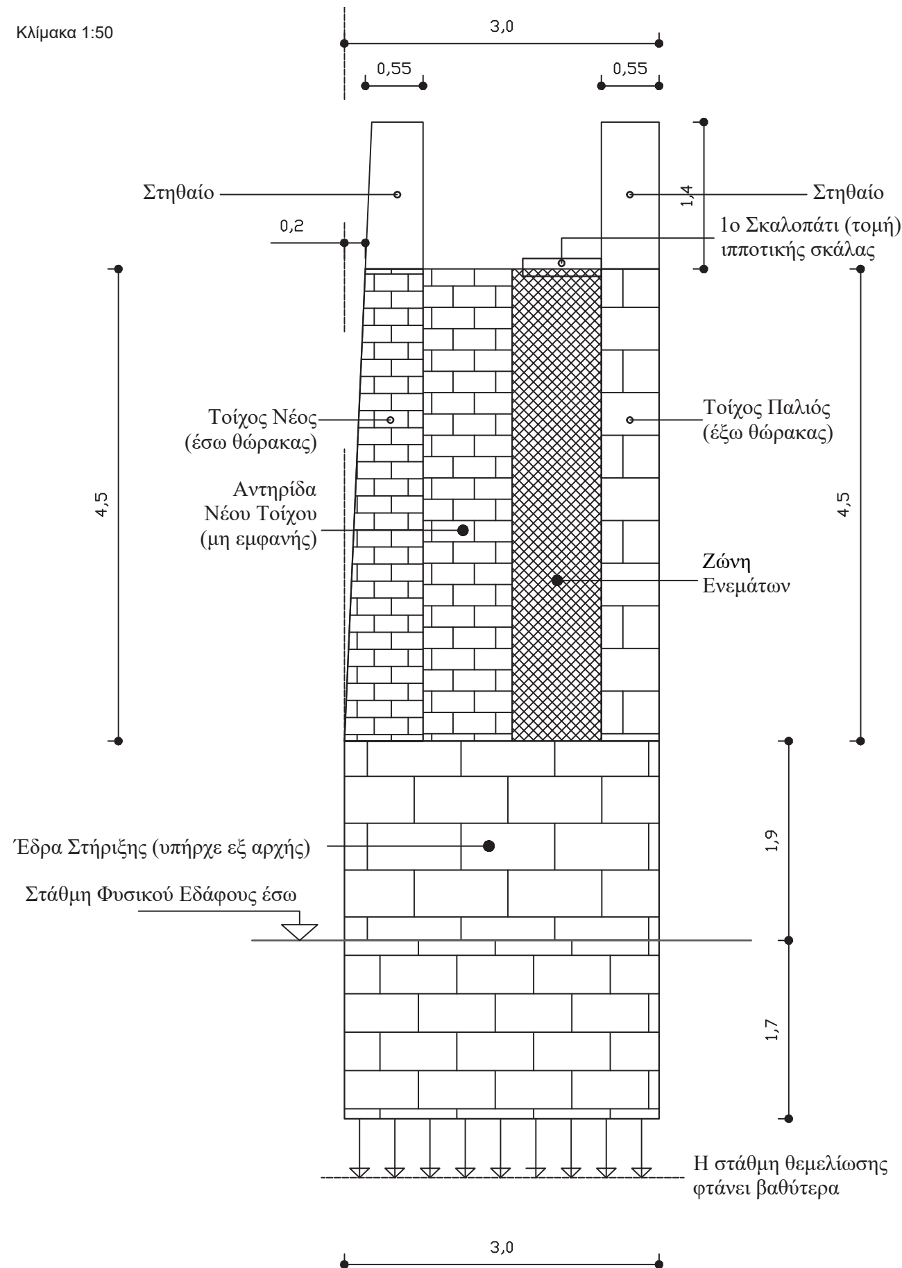
Σχ 3. Σχηματική εγκάρσια τομή
