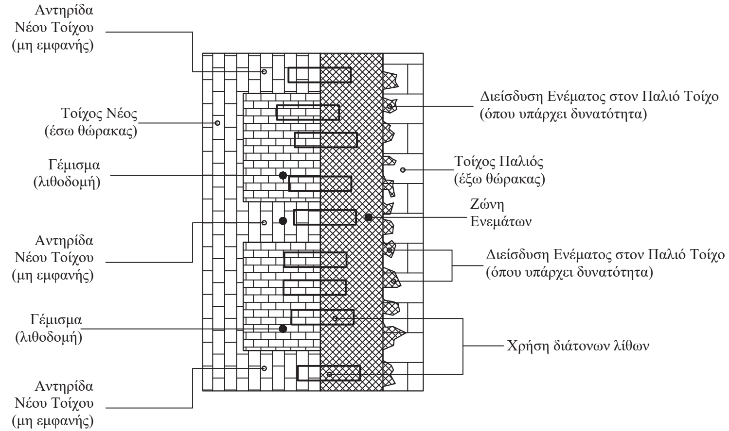
Σχ 6. Σχηματική καθ' ύψος τομή με ορισμένες λεπτομέρειες
