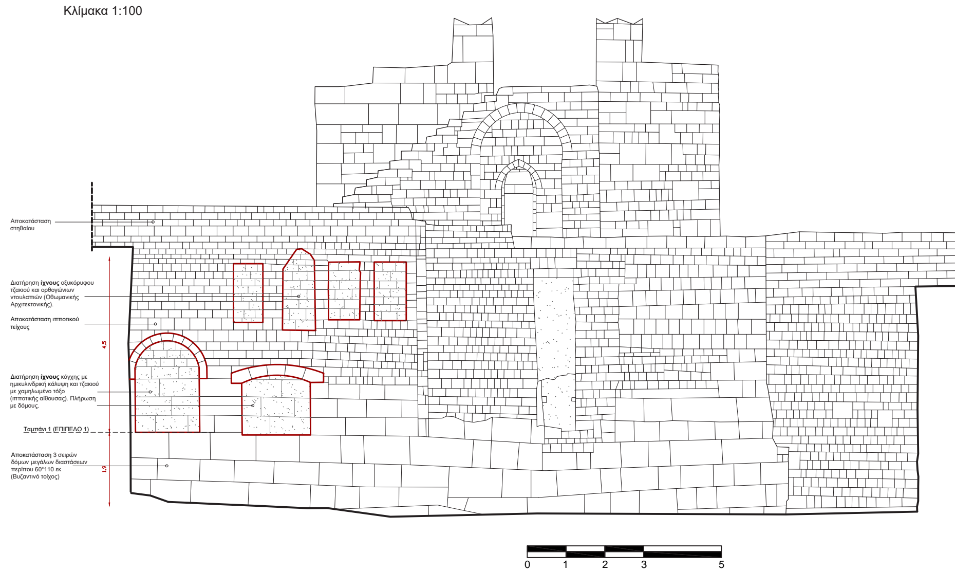
Σχ 2. Εσωτερική όψη του τείχους- πρόταση αποκατάστασης
