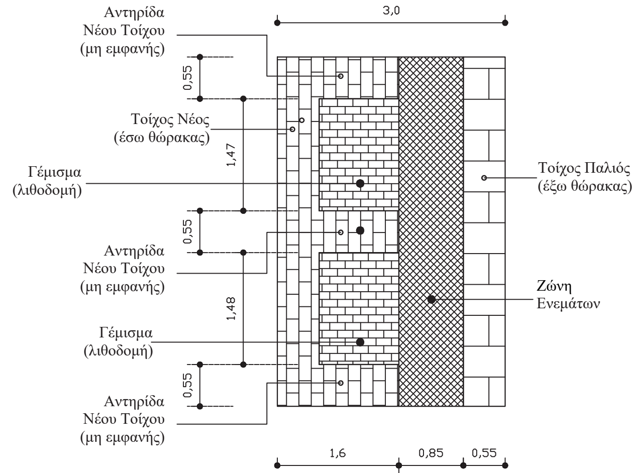
Σχ 5. Σχηματική καθ' ύψος τομή
