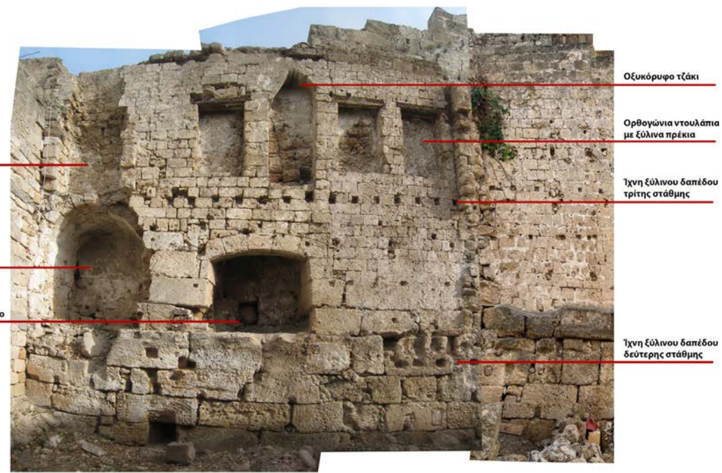
Εικ 5. Φωτογραφική απεικόνιση της εσωτερικής όψης του τείχους ΠΡΙΝ την κατάρρευση. Διακρίνονται τα στοιχεία των διαφορετικών αρχιτεκτονικών φάσεων.
