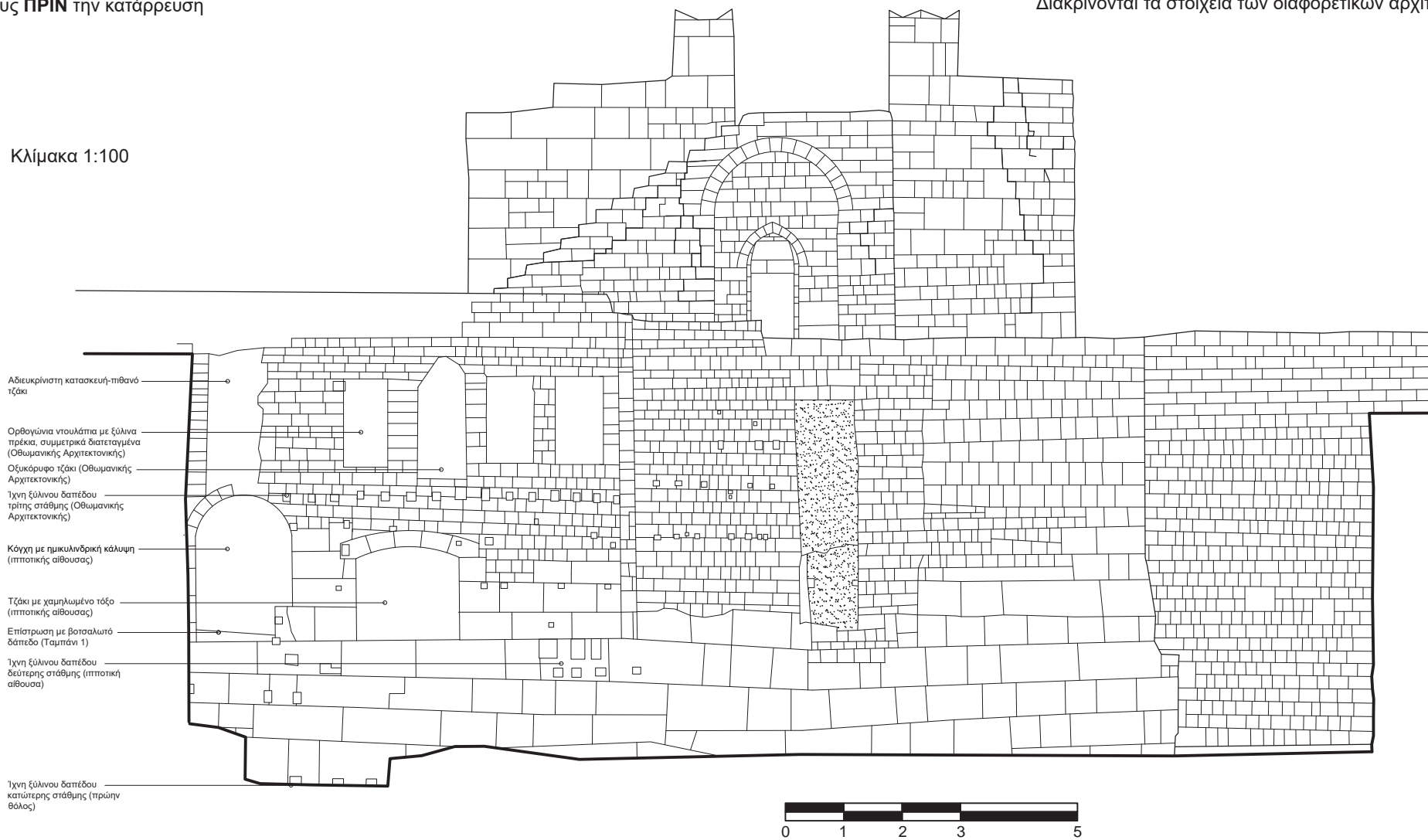
Εικ 6. Εσωτερική όψη του τείχους ΠΡΙΝ την κατάρρευση
