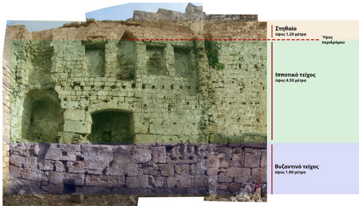
Εικ 4. Σχεδιαγραμματική απεικόνιση τμημάτων του τείχους ΠΡΙΝ την κατάρρευση
